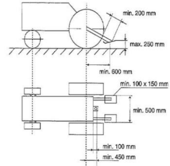
Figuur 14-1: constructie/maatvoering steigerbegrenzer
