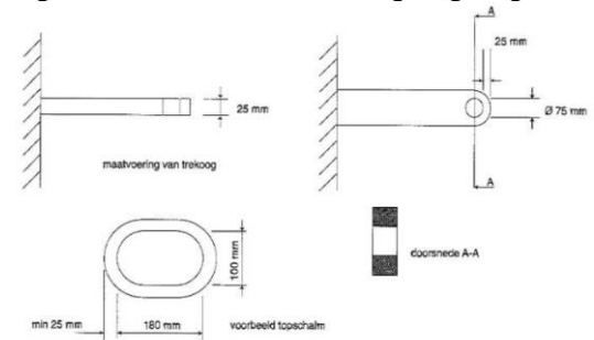
Figuur 14-1: constructie/maatvoering steigerbegrenzer
